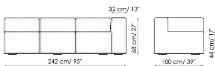
Divano angolare 242 Corner sofa Prof. 100 dx depth right
