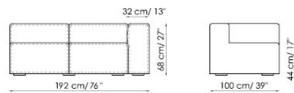
Divano Angolare 192 Corner sofa Prof. 100 dx depth right
